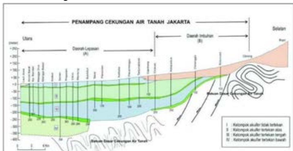
Gambar I.3 Skema Sederhana Penampang Cekungan Air Tanah Jakarta dari Selatan ke Utara
