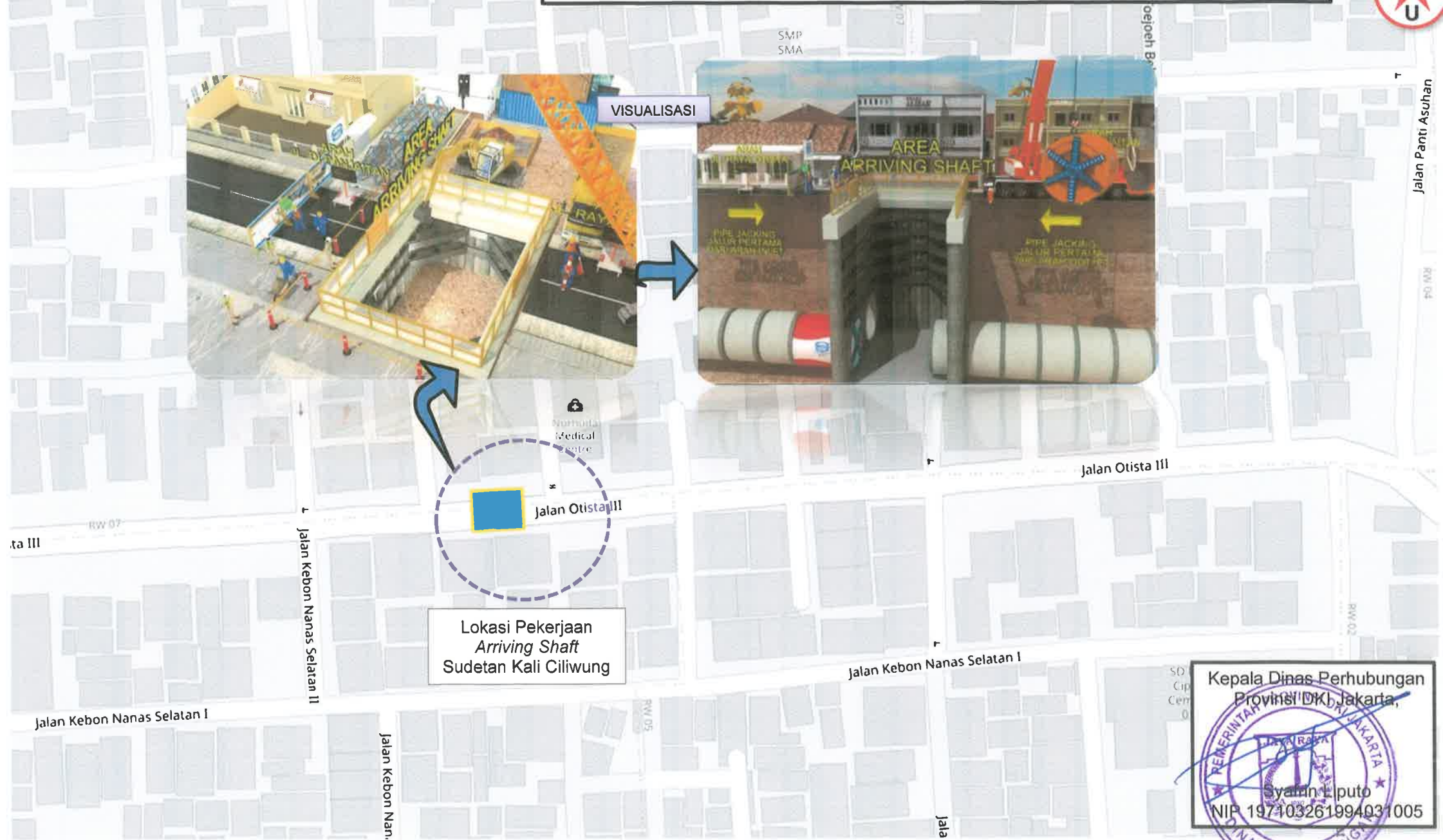
GAMBAR 1 LOKASI PEKERJAAN SUDETAN SUNGAI CILIWUNG DI JALAN OTISTA 3 KOTA ADMINISTRASI JAKARTA TIMUR
